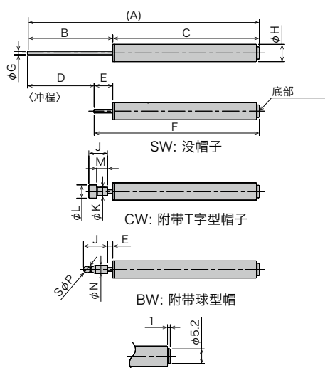
图1 FPD-0725系列的底部形状
