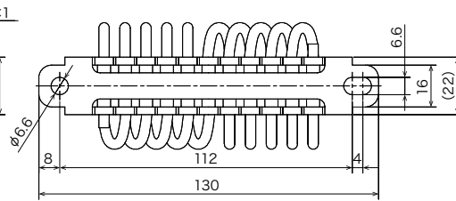
D type (安装部位通孔)
